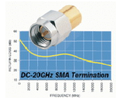
SMA разъем 0 - 20 ГГц
